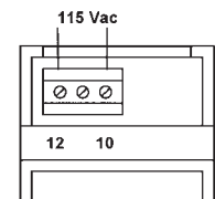
Alimentazione 115 Vac
