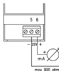
Uscita attiva in corrente 0/4..20 mA
