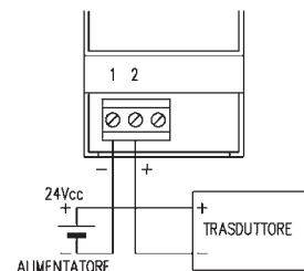
Ingresso passivo in corrente 0/4..20 mA
