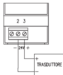
Ingresso attivo in corrente 0/4..20 mA
