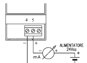
Uscita passiva in corrente 0/4..20 mA
