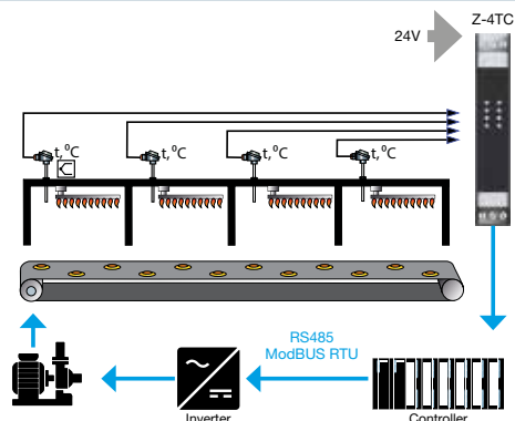
Acquisizione e trasmissione temperature a sistema di controllo in catena chiusa
