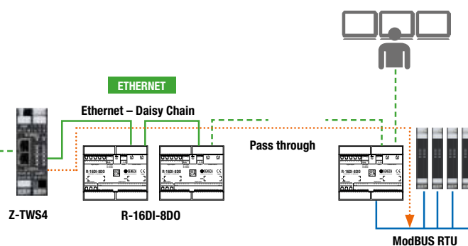
Sistema di imbottigliamento automatico
