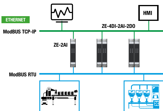
Acquisizione dati su Ethernet
