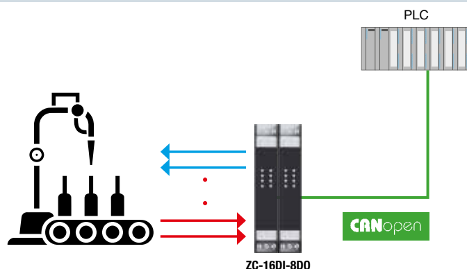
Sistema di imbottigliamento automatico
