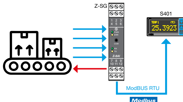
Acquisizione e trasmissione temperature a sistema di controllo in catena chiusa
