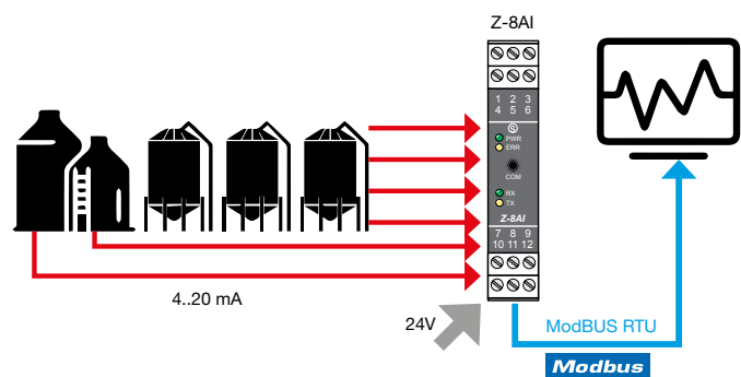
Acquisizione misure di processo e ristrasmissione via ModBUS RTU
