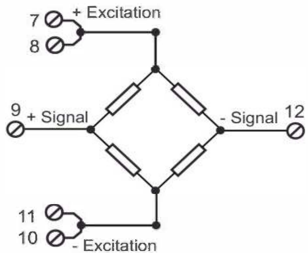
Medición de 4 cables
