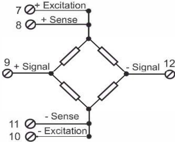
Medición de 6 cables
